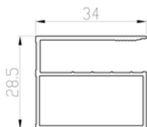
Profilo a muro
