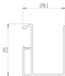
Profilo a muro
