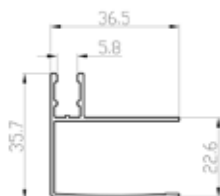
Profilo angolare lato fisso
