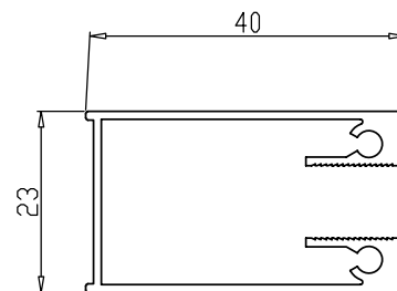
Profilo a muro lato fisso
