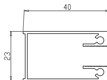
Profilo a muro lato fisso
