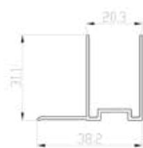
Profilo a parete
